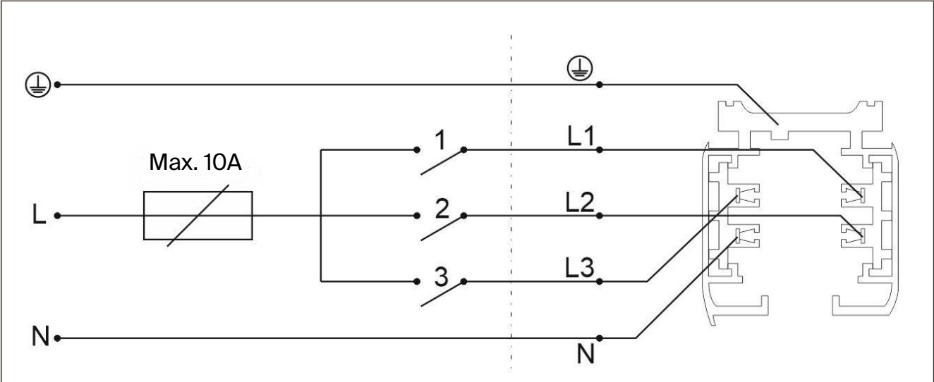
Una línea, en la que el control se divide mediante interruptores monomando.
