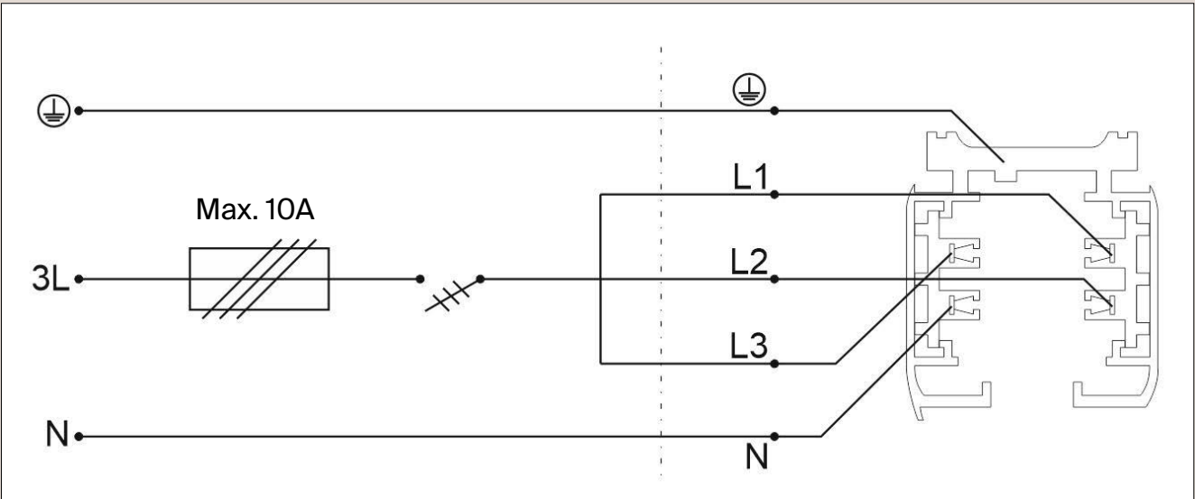
Una línea controlada por un interruptor de tres teclas.
