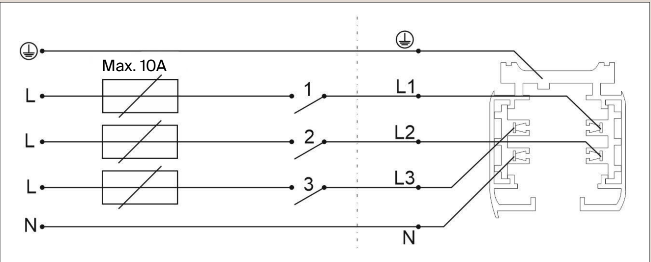
Tres líneas independientes controladas por interruptores de una tecla.
