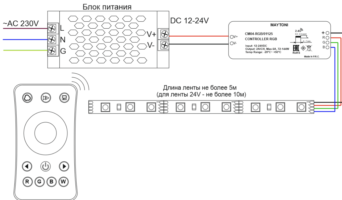
Рис. 1 схема подключения контроллера
