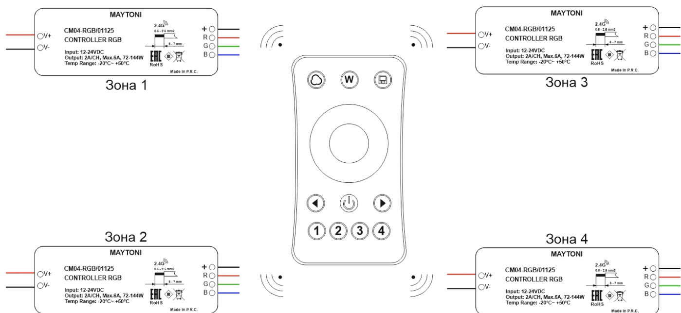
Рис. 3 разветвленная система с многозонным пультом управления
